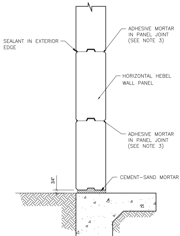
ELEVATION
